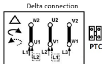
3x400V
