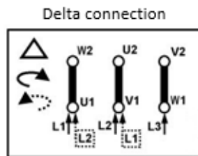
3x400V
