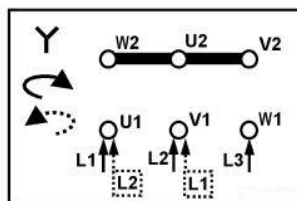
3x400V
