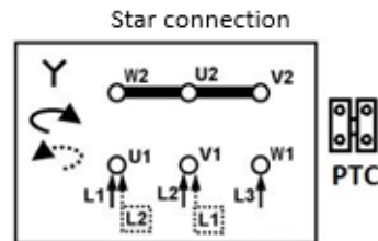
3x400V
