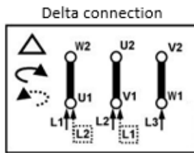
3x230V
