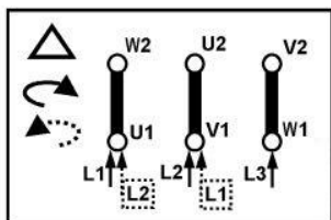
3x230V
